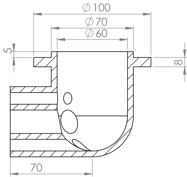
KESIT A-A
