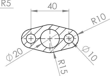
KESIT B-B
