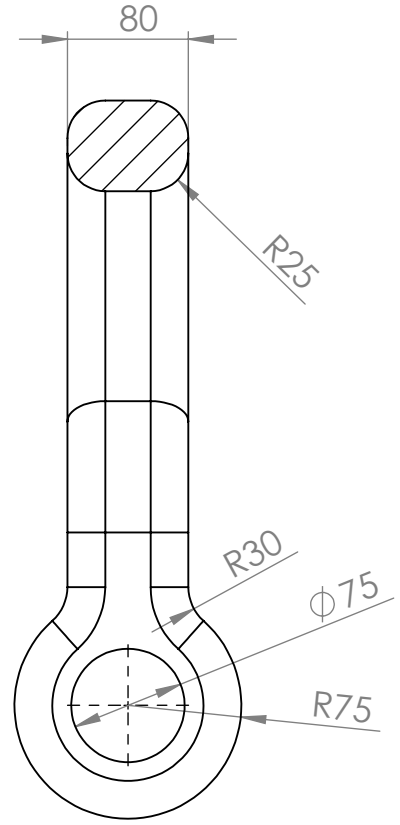
KESIT A-A ÖLÇEK 1 : 5
